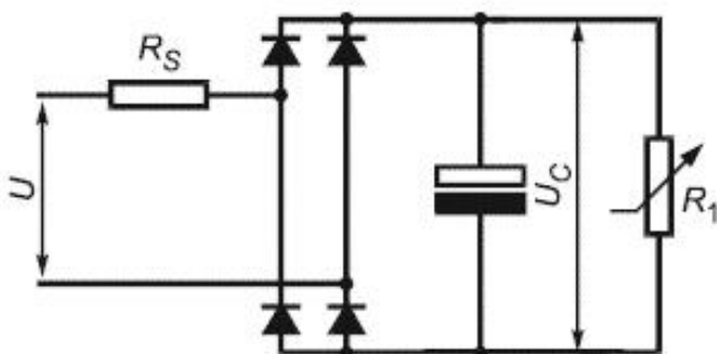
Рисунок М.4 - Эталонная нелинейная нагрузка
