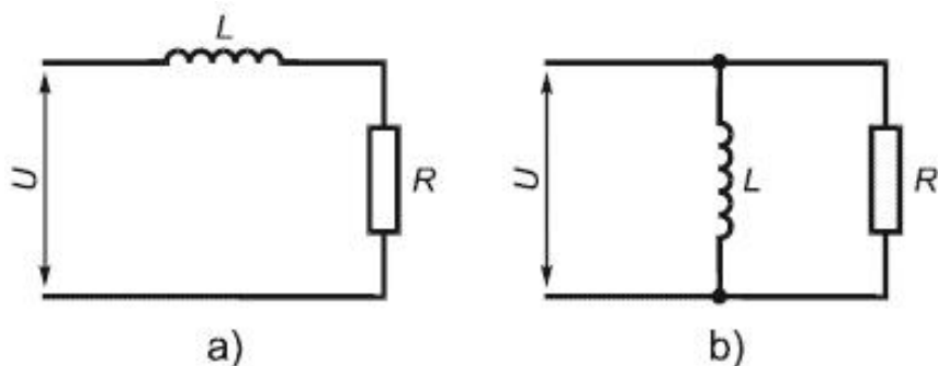
Рисунок М.2 - Эталонная активно-индуктивная нагрузка
