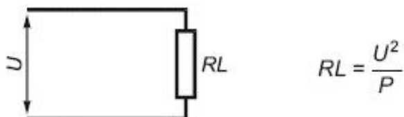
Рисунок М.1 - Эталонная активная нагрузка
